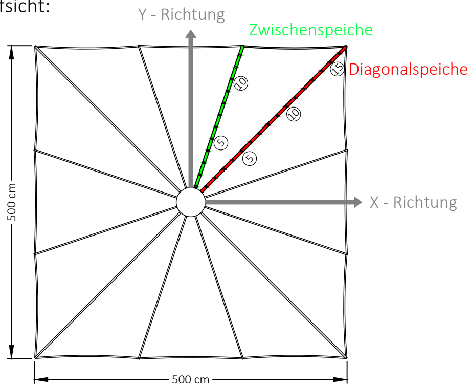
Draufsicht:
