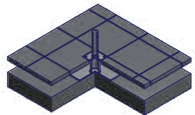
SONDERVERSION NO. 4A AUF BETONDECKE VERANKERT OHNE ENTWÄSSERUNG
