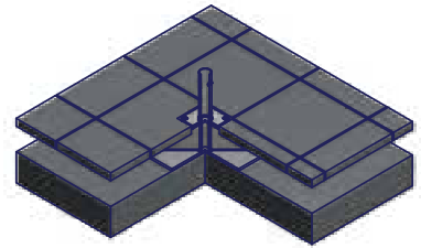
SONDERVERSION NO. 4 MIT KNOTENBLECHEN AUF BETONDECKE VERANKERT OHNE ENTWÄSSERUNG
