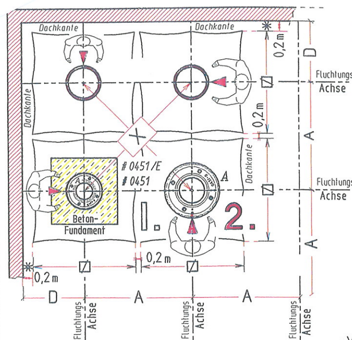
Systemgrundriss
