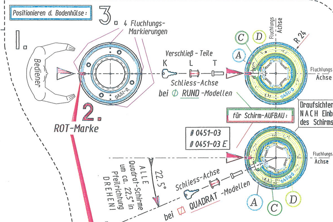
Systemgrundriss
