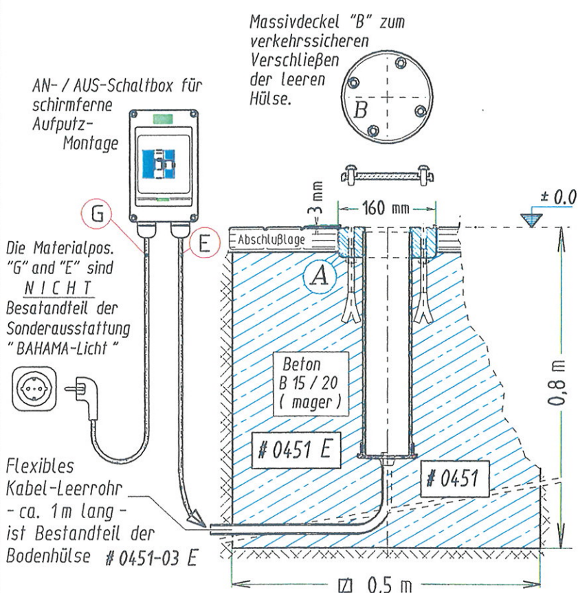
# 0451-.. SCHNITTE
