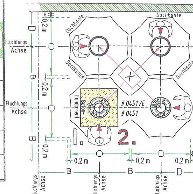
Systemgrundriss
