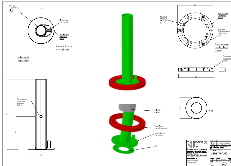
Adapteroberteil (Bodenhülse)
