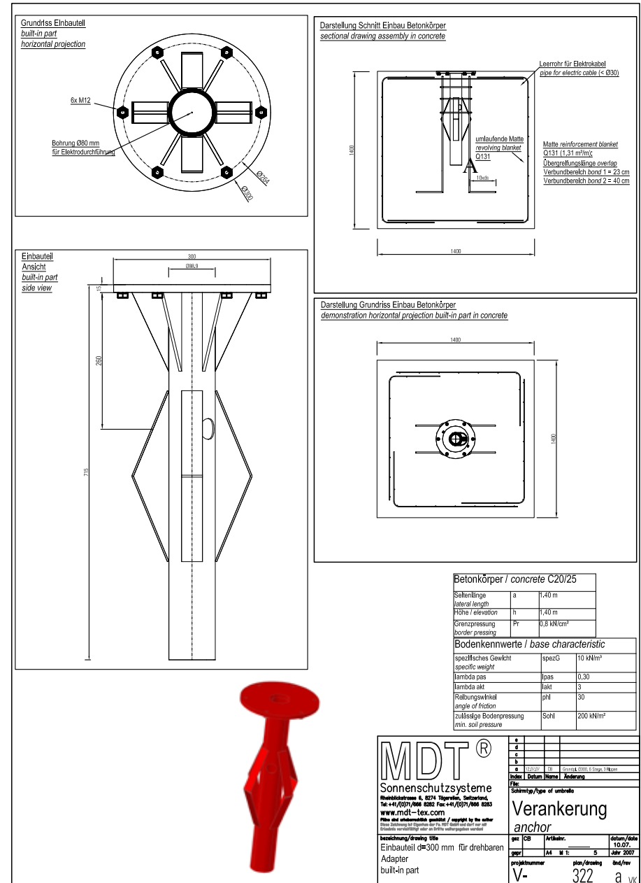
Einbauteil (Bodenhülse)
